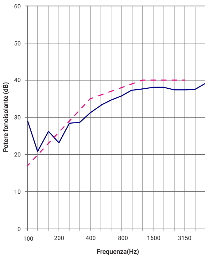
RISULTATI TEST PER PANNELLO DI SPESSORE 18 mm
